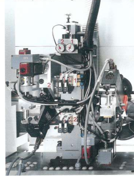
多功能圆弧修边单元 08.0587 Multi-profile milling unit
