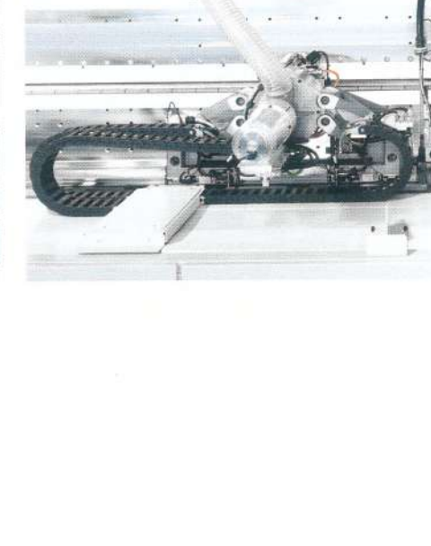
轮廓铣型单元 (KFA) Contour milling unit
