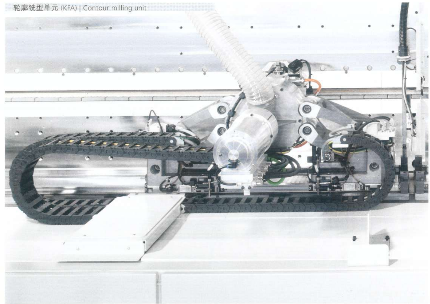
摆臂跟踪单元 (SKF) | Contour trimming unit
