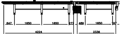
Schema montaggio gambe tappeto 4480 e 2560
