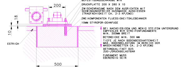
SCHNITT A-A
