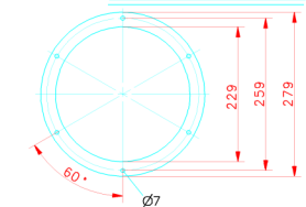
EINZELHEIT "X"
