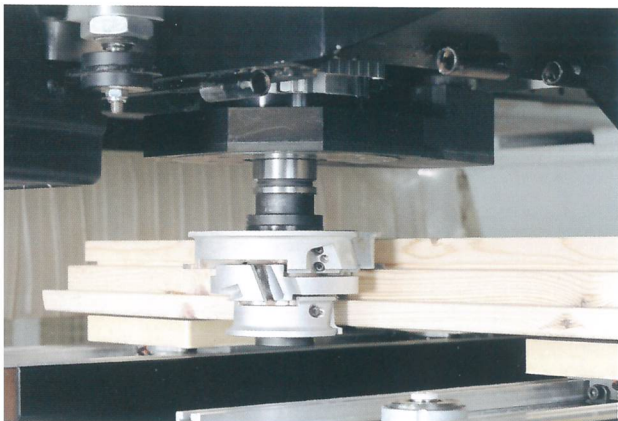
Sbattentatura Formfräsen von Türen und Fenster
