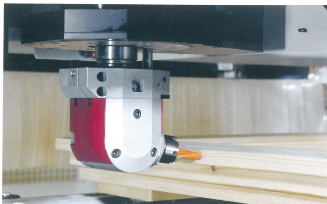
Foratura inclinata per anube. Bohren für Anuba-Bänder
