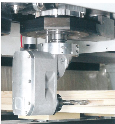
Scasso per serratura Schlosskasten
