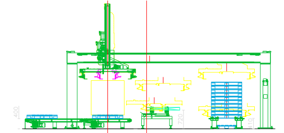
Vista: G-G
