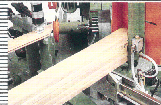
Caricatore automatico - Hopper feed - Chargeur automatique Cargador - Abstellvorrichtung (optional)
