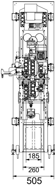
B-B ( 1 : 15 )
