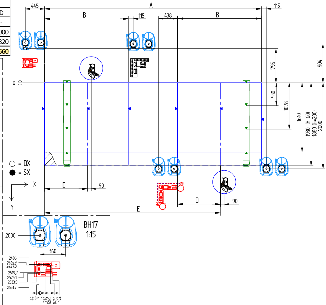
■ Layout Rover B 19XX G configurazione 2 CE
